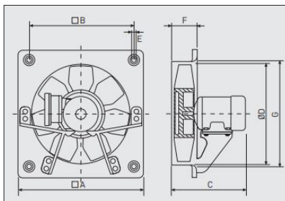
ΔΙΑΣΤΑΣΕΙΣ (mm)
