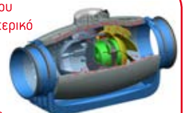
Ειδικά σχεδιασμένο διάτρητο κάσωμα που μέσω των οπών «οδηγεί» τα ηχητικά κύματα στο ειδικό ηχοαπορροφητικό περίβλημα όπου και εκμηδενίζονται.
