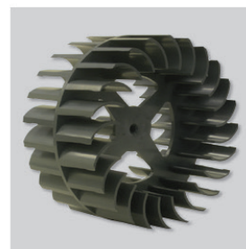
Εμπροσθοκλινή φυγοκεντρική πτερωτή.
