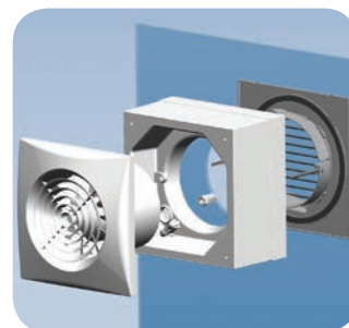
ΣΕΤ ΤΟΠΟΘΕΤΗΣΗΣ ΣΕ ΤΖΑΜΙ
