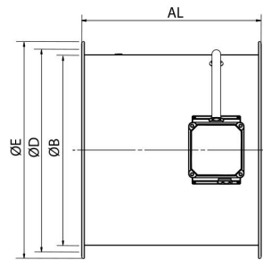
TGT long casing
