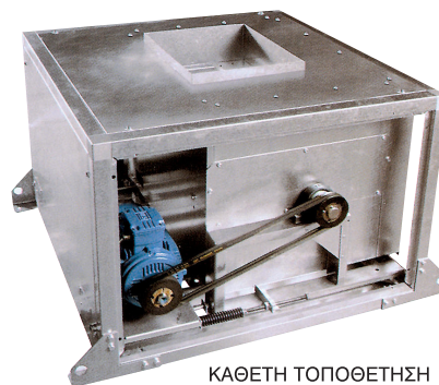
ΚΑΘΕΤΗ ΤΟΠΟΘΕΤΗΣΗ
