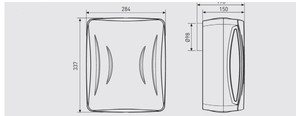
EBB-170 N - 250N
