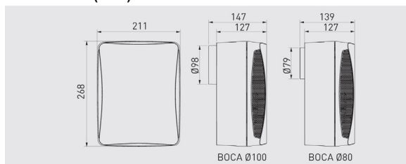
ΔΙΑΣΤΑΣΕΙΣ (mm) EBB-100 N
