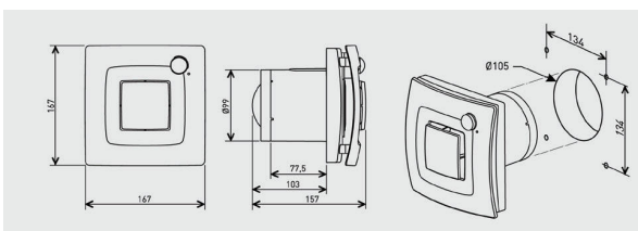
ΔΙΑΣΤΑΣΕΙΣ (mm)
