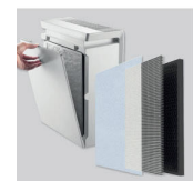
Φίλτρο Ινών Φίλτρο HEPA Φίλτρο ενεργού άνθρακα
