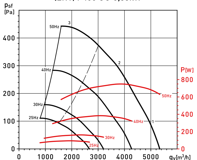
ILHT/4-400 CC 0,55kW
