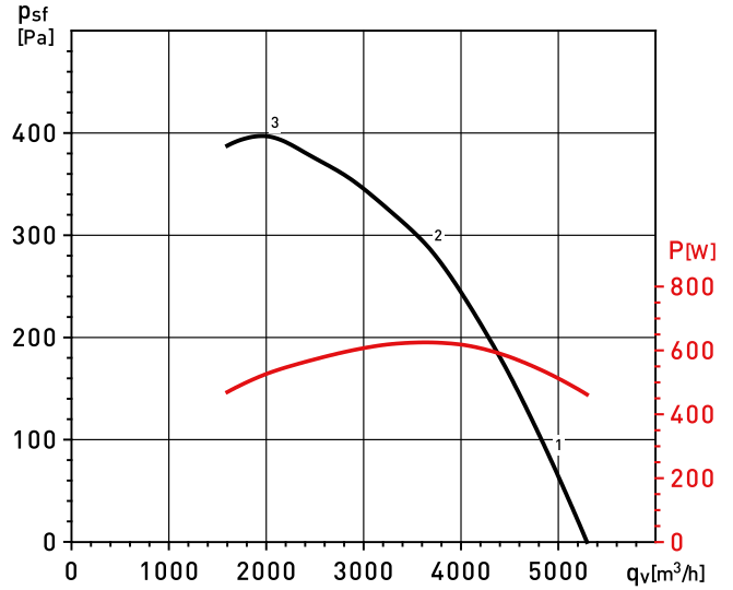
ILHB/4-400 MV 0,55kW
