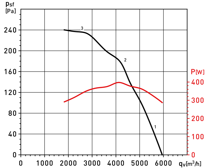
ILHB/6-500 MV 0,37kW
