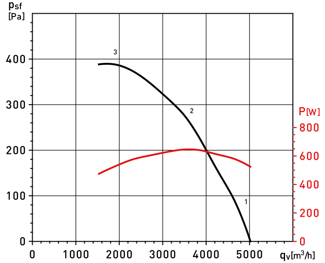
ILHB/4-400 CC 0,55kW
