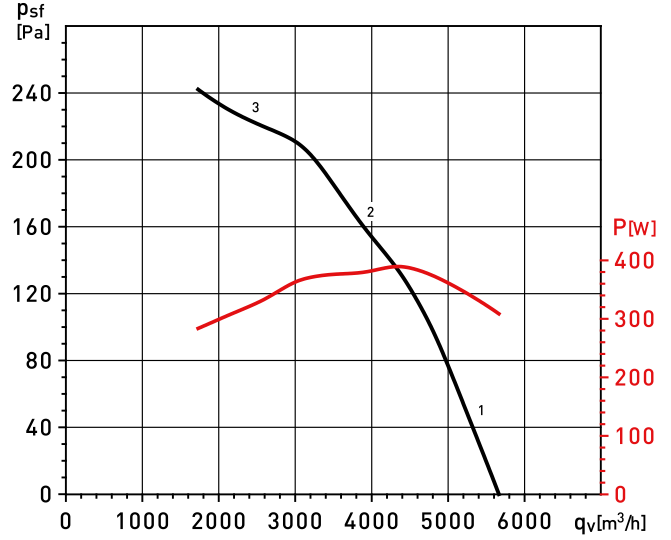
ILHB/6-500 CC 0,37kW
