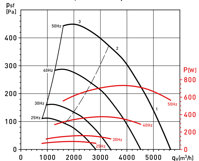
ILHT/4-400 MV 0,55kW
