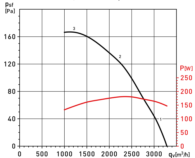
ILHB/6-400 CC 0,25kW
